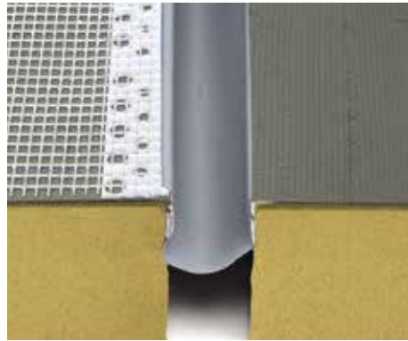
Kalekim Dilatasyon Profili
